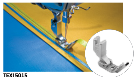
TEXI 5015 Fuß mit zentral Bandzuführung 4.8mm
