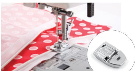
TEXI 1015 MATIC Reißverschlussfuß verdeckt
